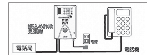
通話録音装置設置図
